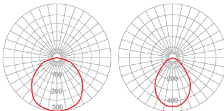
Рисунок 2. Кривые силы света
