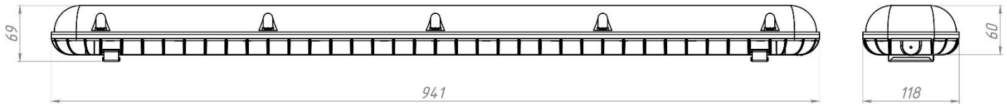
Рисунок 1. Внешний вид на вариант светильника.
