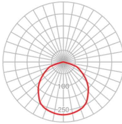
Рисунок 2. Кривые силы света
