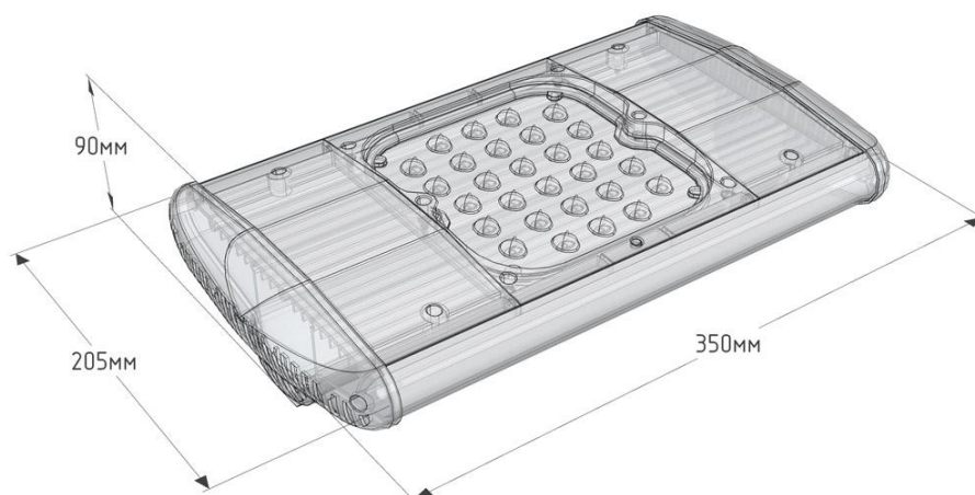
Рисунок 1. Внешний вид на вариант светильника.
