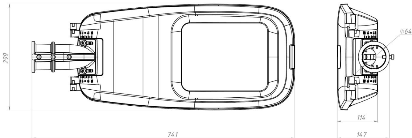
Рисунок 1. Внешний вид на вариант светильника.
