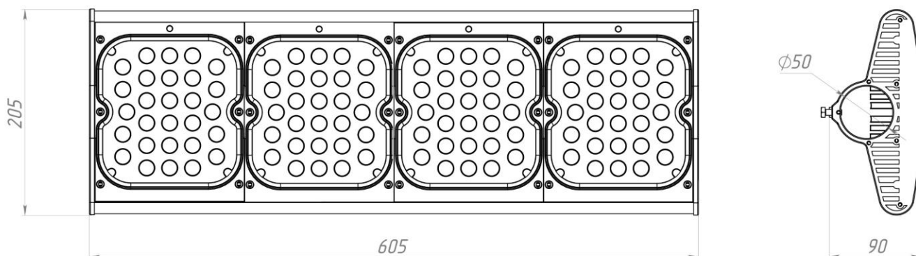
Рисунок 1. Внешний вид на вариант светильника.
