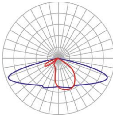
Рисунок 2. Кривые силы света
