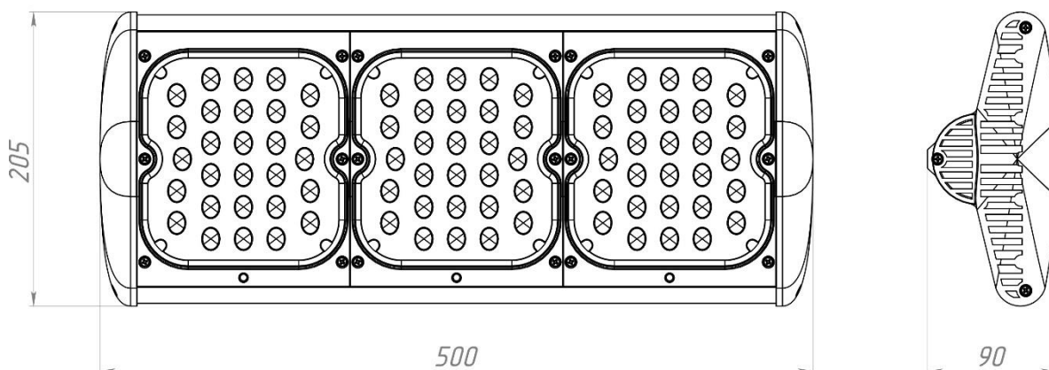
Рисунок 1. Внешний вид на вариант светильника.
