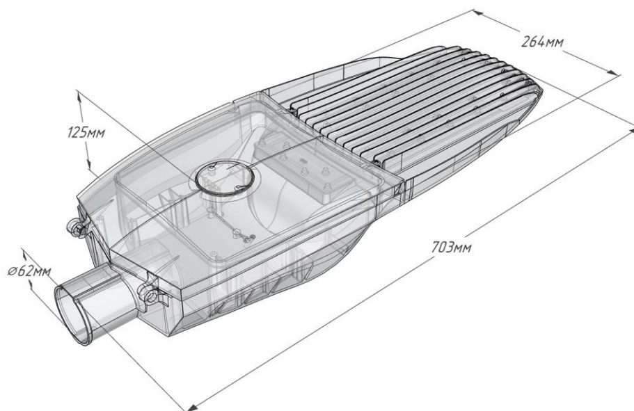
Рисунок 1. Внешний вид на вариант светильника.
