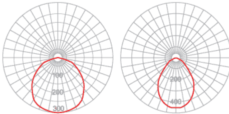
Рисунок 2. Кривые силы света
