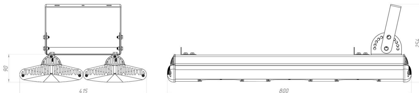
Рисунок 1. Внешний вид на вариант светильника.
