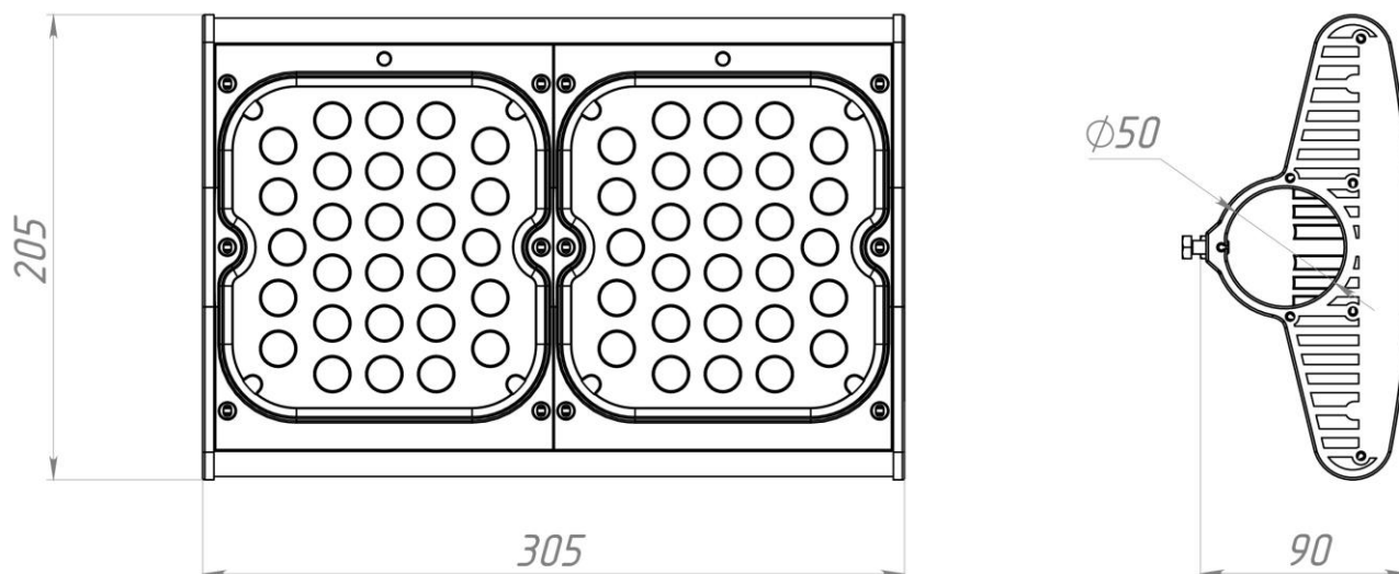
Рисунок 1. Внешний вид на вариант светильника.
