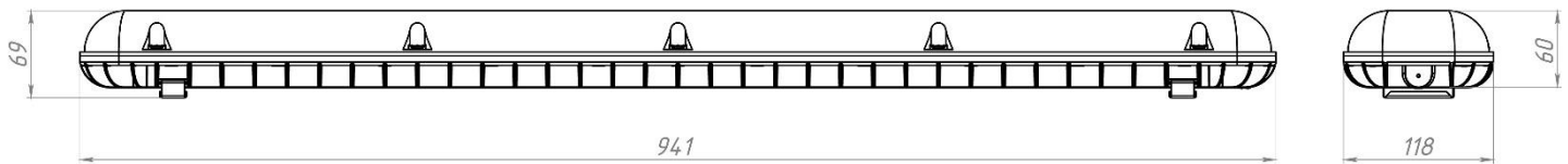
Рисунок 1. Внешний вид на вариант светильника.
